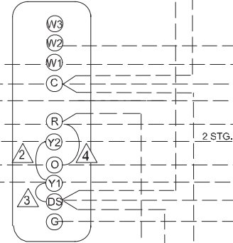
INDOOR UNIT 24 VOLT TERMINAL STRIP
